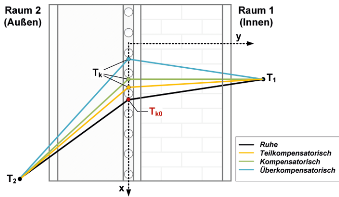
Bild 6. Schematische Änderung der Temperatur in der Heizebene ( T_k ) durch den Betrieb der aWT und Zuordnung der Betriebsituationen
