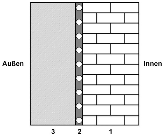
Bild 1. Vereinfachter schematischer Wandaufbau der aWT, mit Bestandswand (1), thermisch aktive Schicht (2) und WDVS (3)
