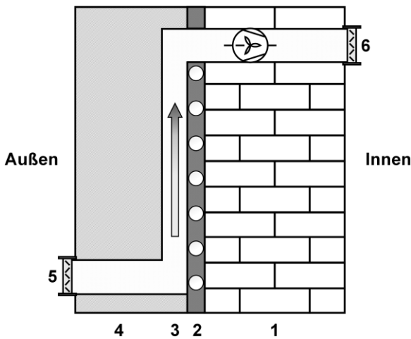
Bild 2. Vereinfachter schematischer Wandaufbau der aLT, mit Bestandswand (1), thermisch aktiver Schicht (2), Luftspalt (3), WDVS (4), Lufterinlass (5) und Luftauslass (6) jeweils mit Klappe
