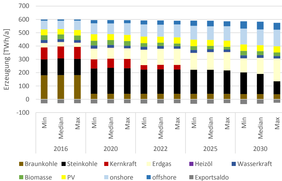
Abbildung 27 Entwicklung der Stromerzeugung nach Technologien im Ziel-Szenario bei minimalem, mittlerem und maximalen CO 2 -Preisfad
