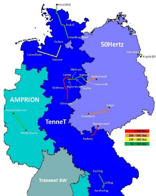
Abbildung 11 Strombedingte Redispatch-Maßnahmen 2012 (am stärksten betroffene Netzelemente) Quelle: in BNetzA 2014d, S.60
