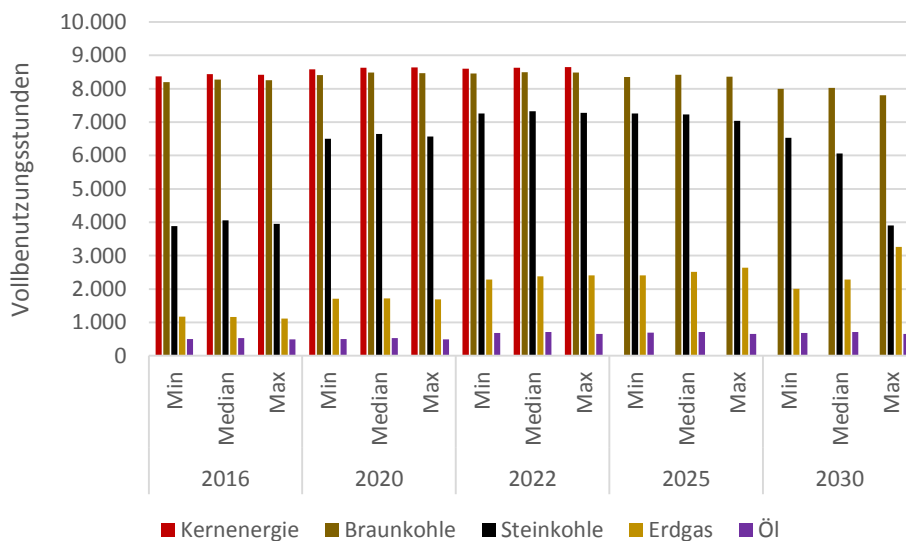
Abbildung 28 Entwicklung der Vbh im Ziel-Szenario bei niedriger, mittlerer und hoher Preisentwicklung bei minimalem, mittlerem und maximalen CO 2 -Preisfad
