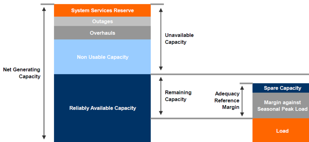
Abbildung 9 Schematische Beschreibung der Leistungsbilanz nach ENTSO-E Quelle ENTSO-E 2014 (S. 136)
