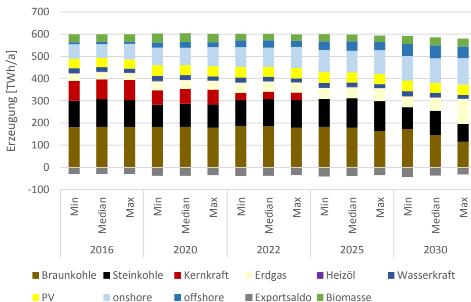
Abbildung 15 Entwicklung der Stromerzeugung nach Technologien im Referenzszenario bei minimalem, mittlerem und maximalem CO 2 -Preisfad
